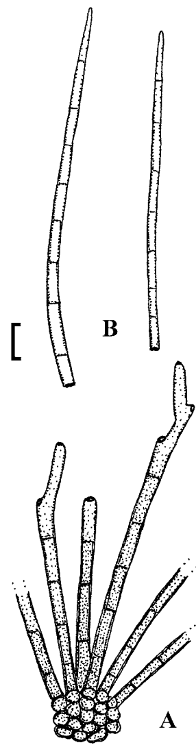
Fig. 15. Cercospora asplenii (HBG, holotype). A. Conidiophore fascicle. B. Conidia. Bar = 10 \mu m.
