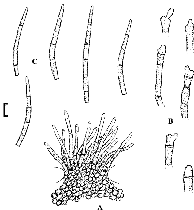
Fig. 63. Pseudocercospora juniperi (NY, holotype). A. Conidiophore fascicle. B. Conidiophores. C. Conidia. Bar = 10 \mu m.
