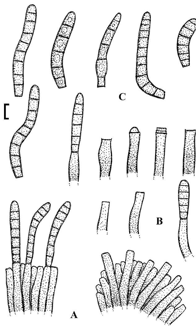
Fig. 67. Pseudocercospora thujina (BPI 404872). A. Conidiophore fascicles. B. Conidiophores. C. Conidia. Bar = 10 \mu\text{m} .
