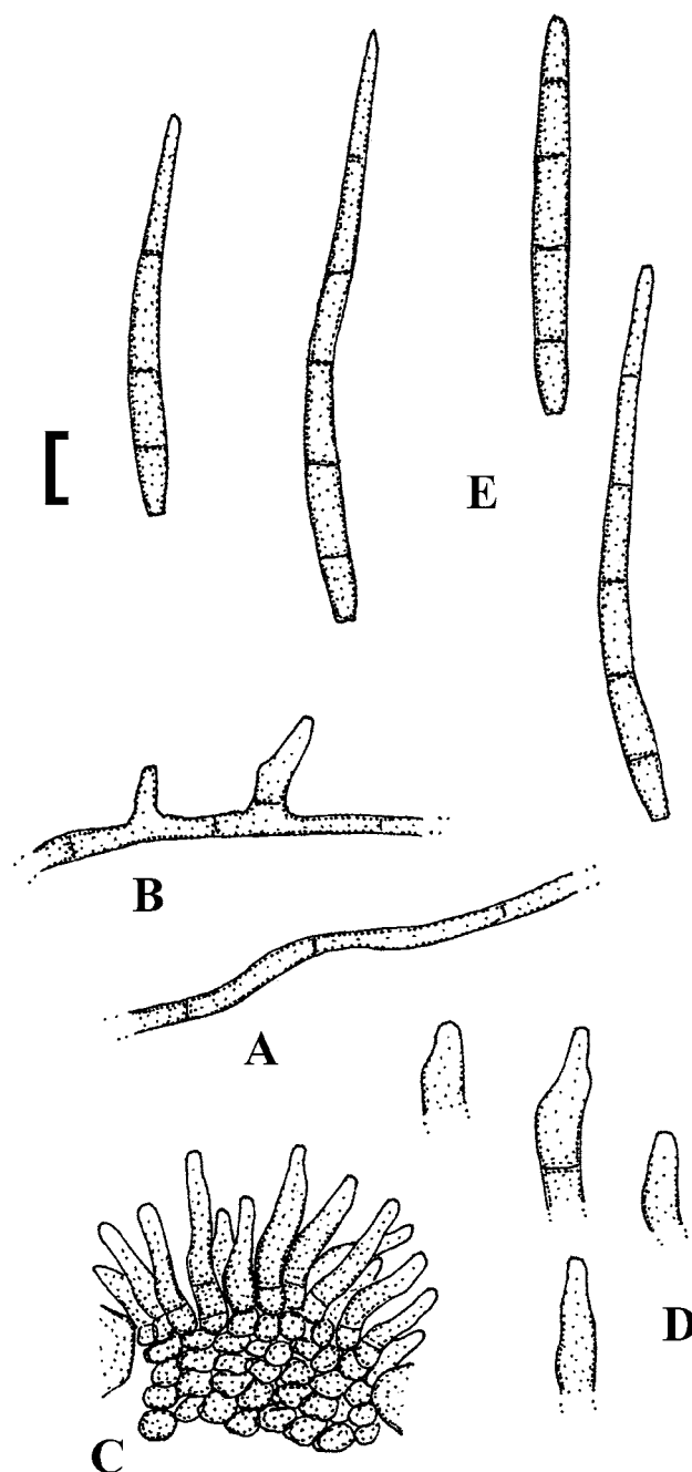
Fig. 50. Pseudocercospora pteridicola (HMAS 59158). A. Superficial hypha. B. Solitary conidiophores arising from a superficial hypha. C. Conidiophore fascicle. D. Conidiophores. E. Conidia. Bar = 10 µm.
