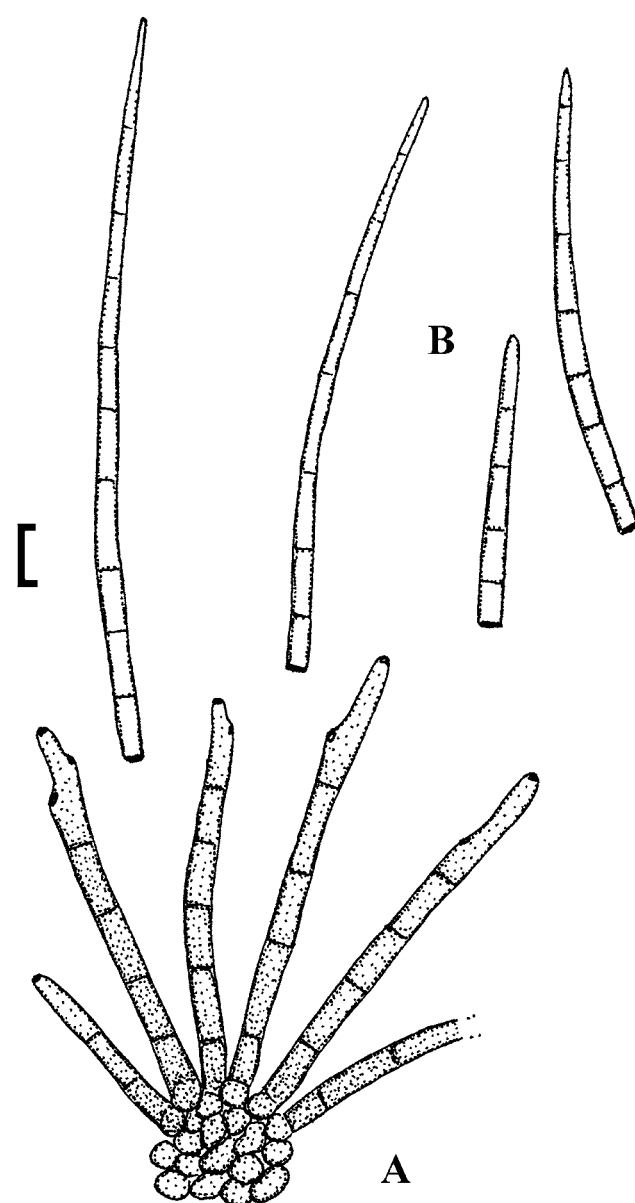
Fig. 18. Cercospora cyclosori (K(M) IMI 312082). A. Conidiophore fascicle. B. Conidia. Bar = 10 \mu m.
