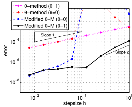
(d) Error for \mathbb{E}(X_{[2]}^2) . Stiff case \alpha = 25 .
