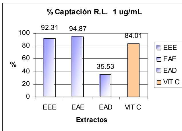
Gráfico N° 3: Porcentaje de captación de radicales Libres a 1 ug/mL
