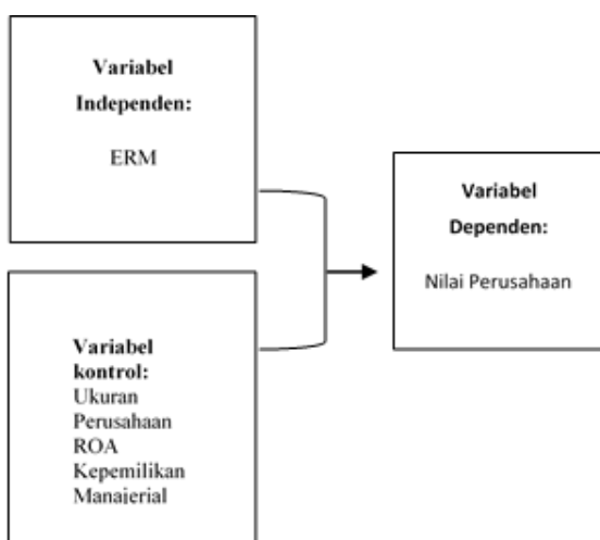
Gambar 1. Kerangka Konseptual
