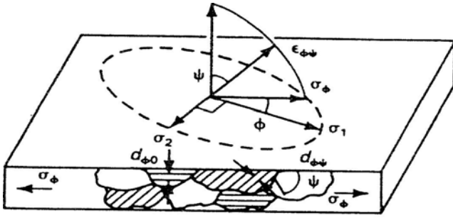
Fig. 2 -Plane-stress elastic model
