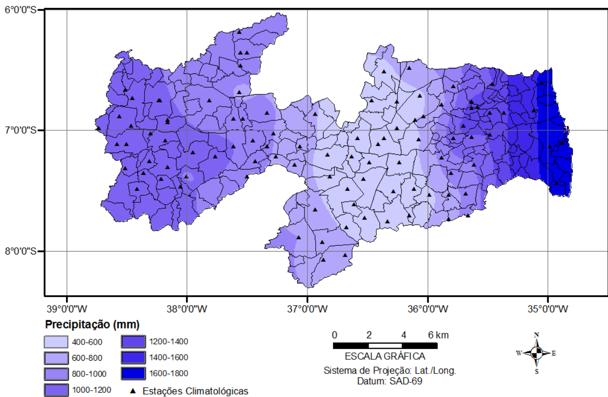
Figura 7 – Localização das estações climatológicas utilizadas e a precipitação total para o Estado da Paraíba.
