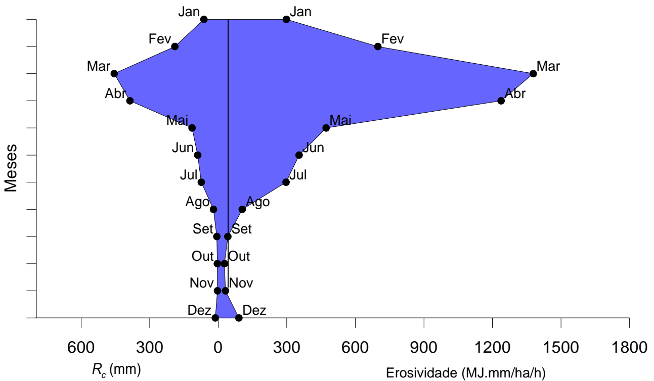
Figura 4 – Relação entre erosividade da chuva e o coeficiente de chuva para todas as estações climáticas utilizadas no estudo.
