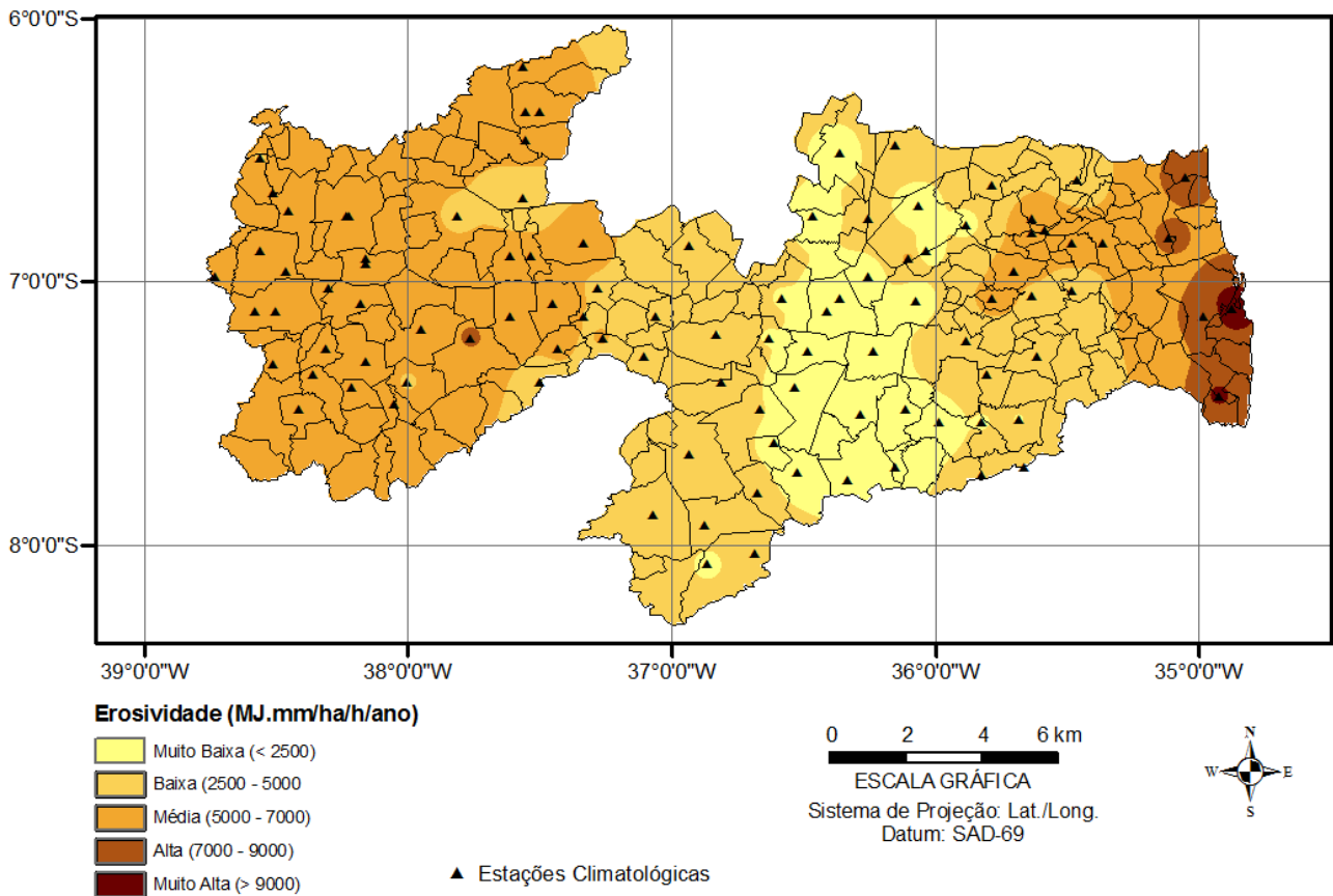
Figura 10 – Áreas isoerosivas obtidas a partir do método de Krigagem.
