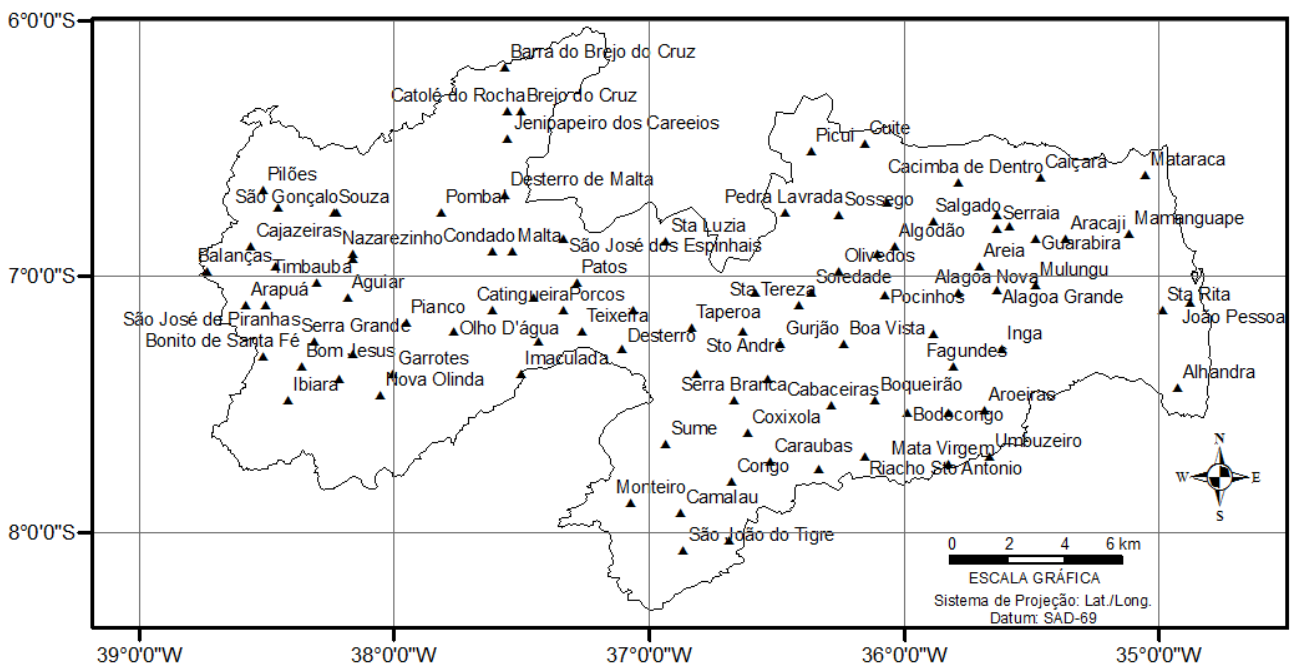
Figura 2 – Distribuição espacial das estações climatológicas utilizadas
