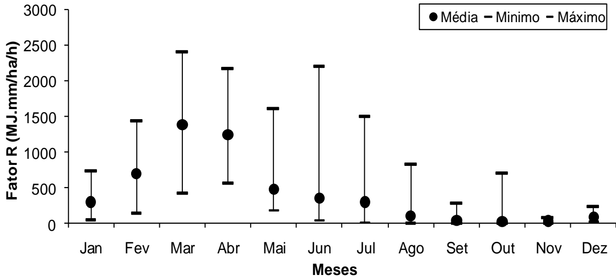
Figura 3 – Distribuição média mensal do fator de erosividade para a Paraíba, no período de 1910 a 1990.
