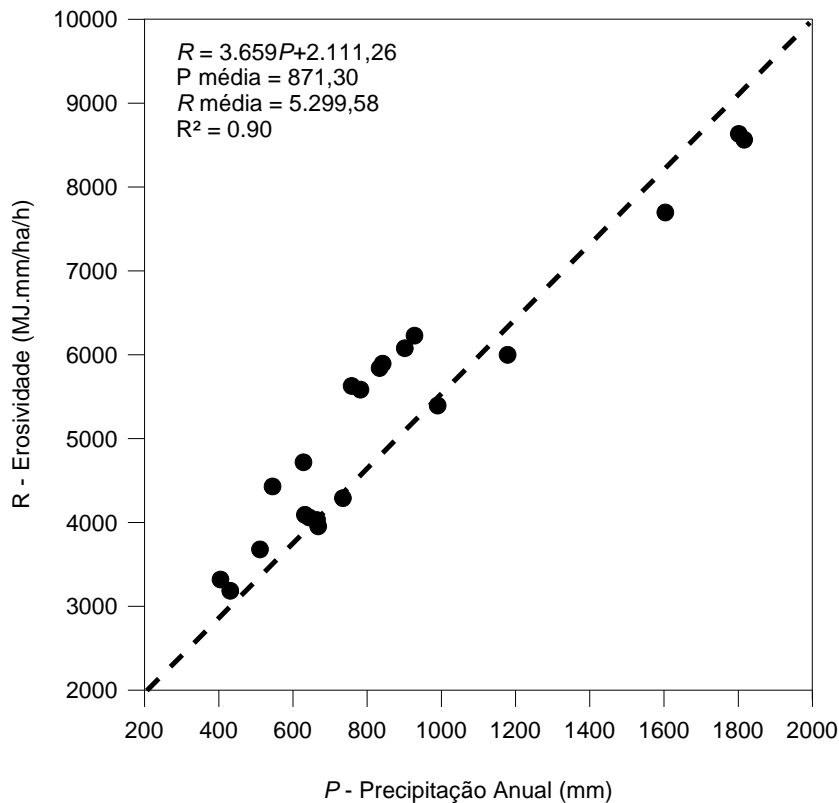
Figura 9 – Relação entre precipitação total anual e erosividade anual, para cada microrregião do Estado da Paraíba.
