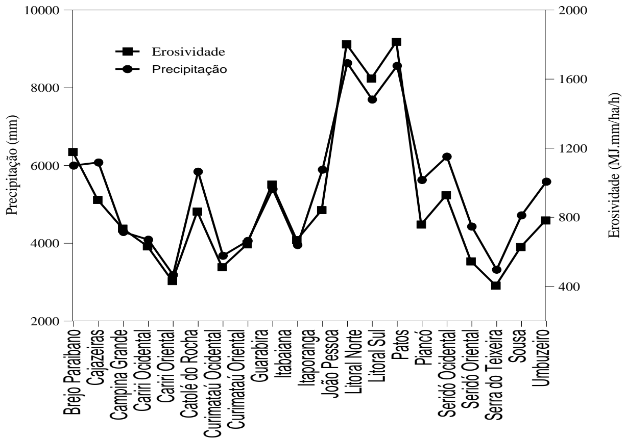
Figura 6 – Precipitações médias anuais para as microrregiões do Estado da Paraíba.
