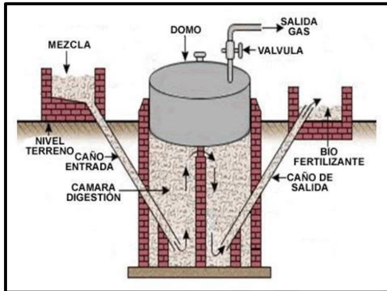
FIGURA 8. Modelo de un biodigestor
