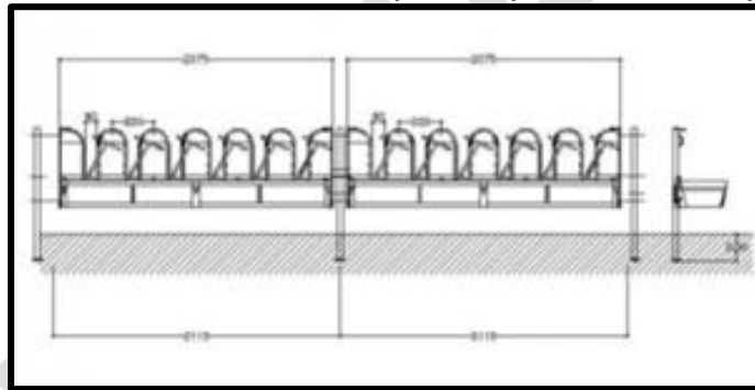
FIGURA 4. Instalación para explotación de caprinos
