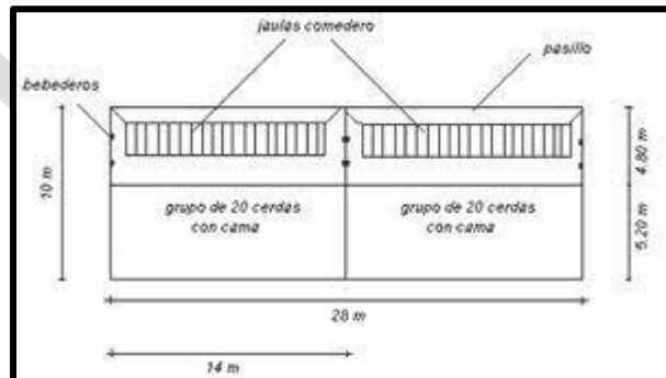
FIGURA 3. Instalación para explotación de cerdos
