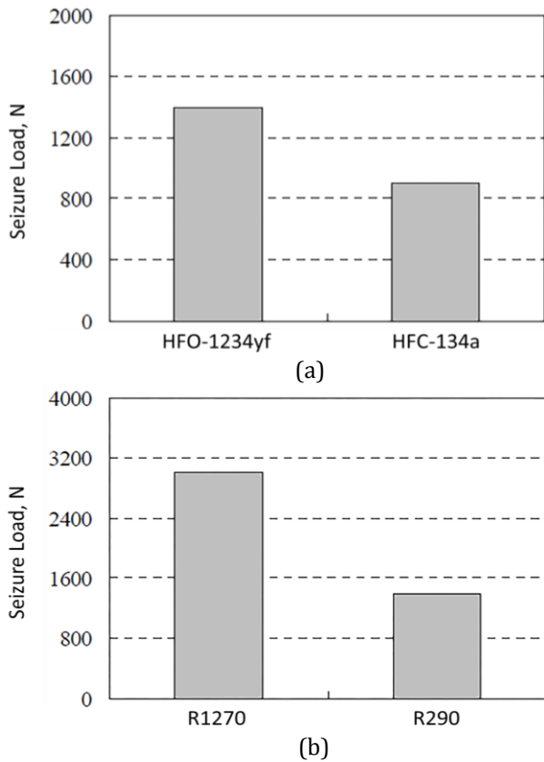
Fig. 16. Seizure load [109].
